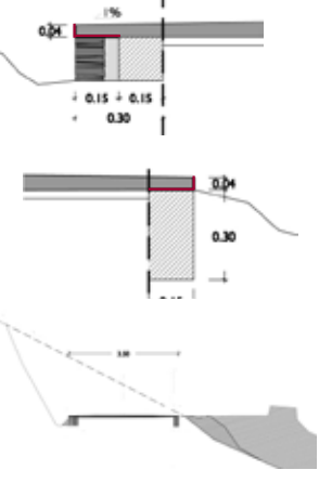
Seccions tipus de la vialitat restaurada
